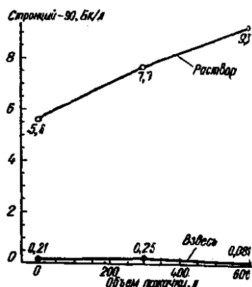
Рис. 4. Изменение содержания стронция-90 в скважине К-9 в ходе прокачки 8.09.93 г.
