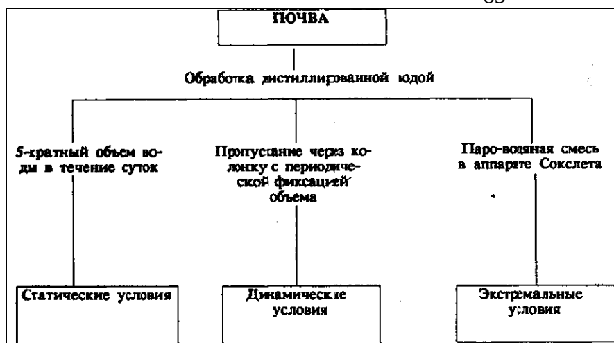
Рис. 1 Схема выделения водорастворимых форм РН в различных условиях
