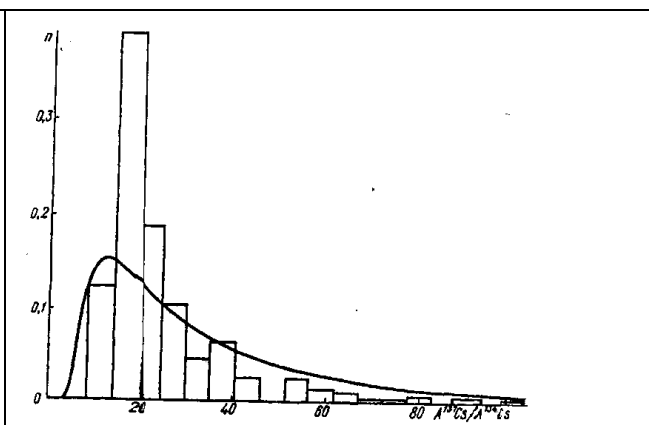
Рис. 3. Логарифмически нормальное распределение отношений активности ^{137}\text{Cs} к активности ^{134}\text{Cs} (на сентябрь 1992 г.)
