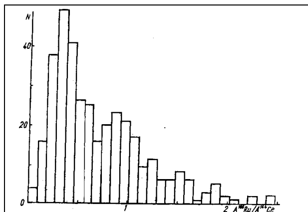
Рис. 2. Гистограмма отношений активности ^{106}\text{Ru} к активности ^{144}\text{Ce} (на сентябрь 1992 г.)
